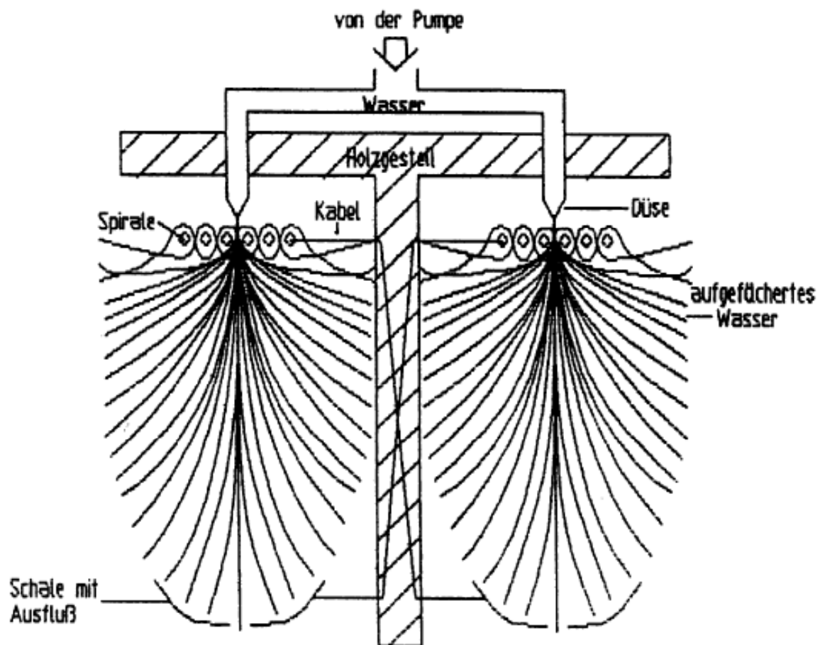
Bild 1: Querschnitt des Aufbaus (vereinfacht)
